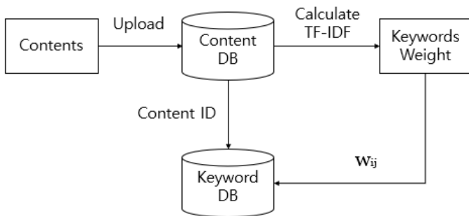
[그림1] 강좌의 키워드 처리를 위한 모델 구조
