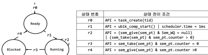
그림 4. 세마포어 상태 기계
