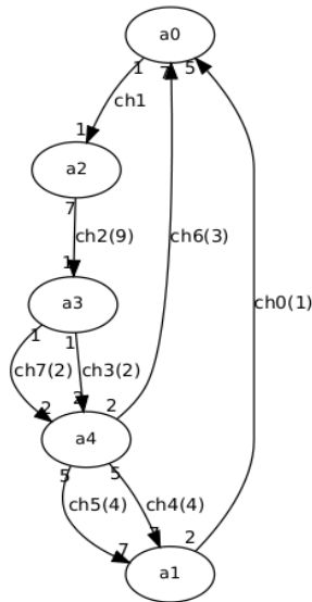
그림 6. 랜덤 생성된 SDF 그래프 예시
