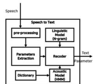
그림 4. Speech-to-Text Layer 구조도
