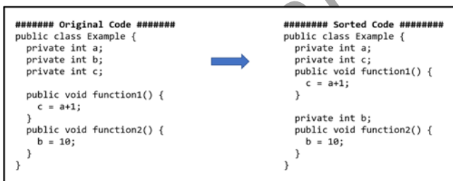
그림 2. 소스 코드 정렬 결과 예
