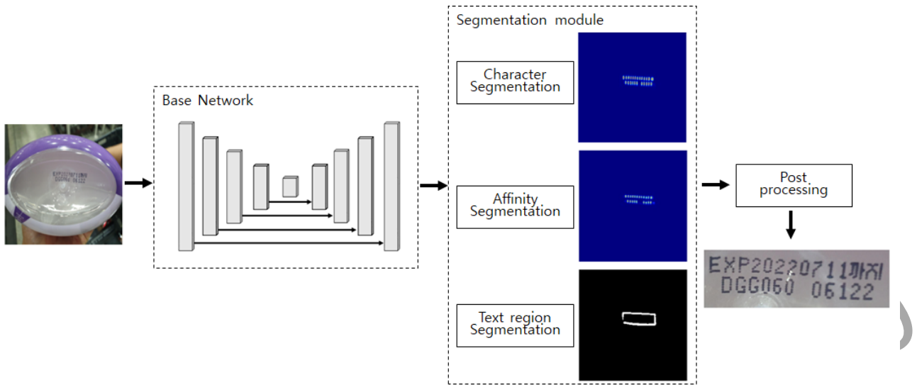
그림 3: 글자 기반 세그멘테이션 검출 모델 구조.
