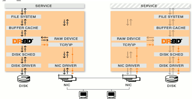
그림 2. DRBD Architecture
