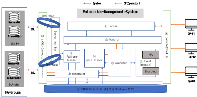
그림 5. System Architecture
