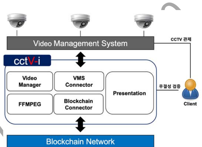
그림 1 CCTV 블록체인 플랫폼 개요
