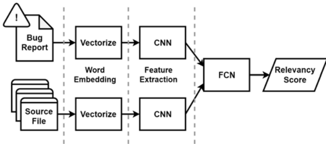
그림 1. CNN 기반 버그 추적 모델
