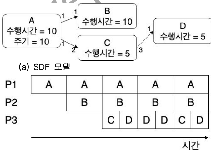
(b) (a)에 대한 매핑/스케줄링
