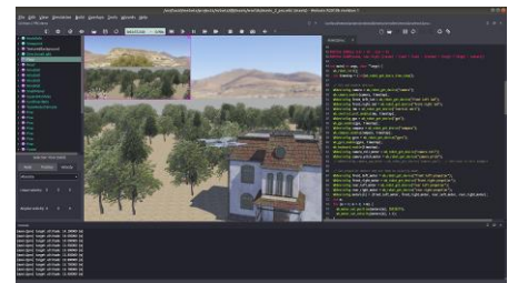
(i) Webots
