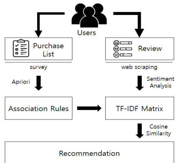
그림2. 시스템 프로세스
