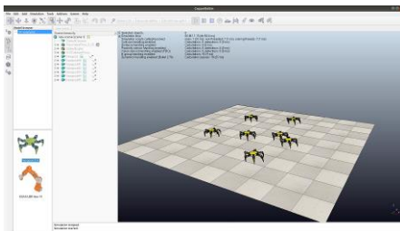
(j) CoppeliaSim
