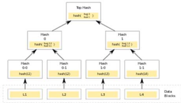
그림 2. Merkle Tree
